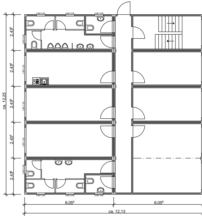
Grundriss-Erdgeschoss
